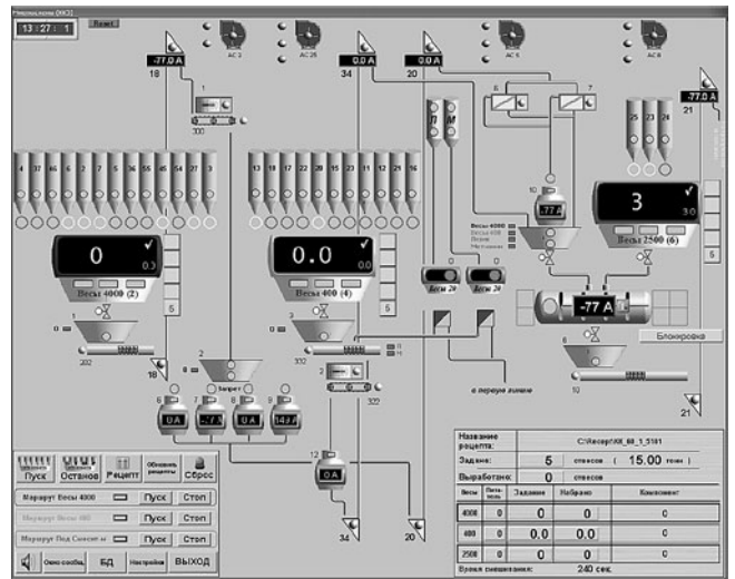
Рис. 2. Мнемосхема технологического процесса
