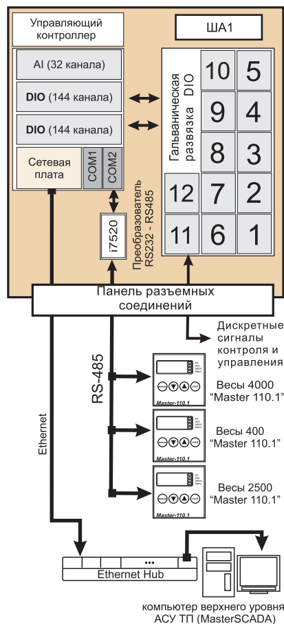
Рис. 1. Структура системы
